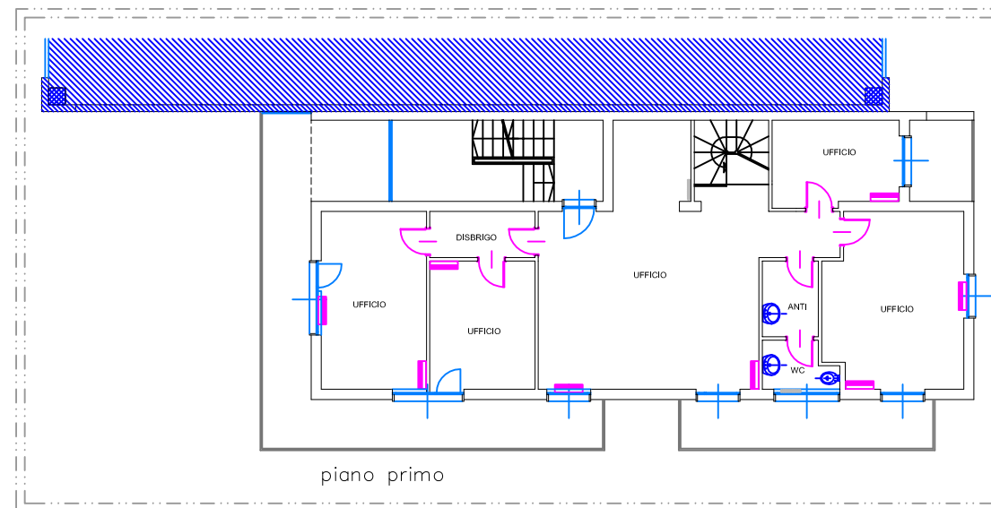
UFFICI MISIONE - PIANO PRIMO
