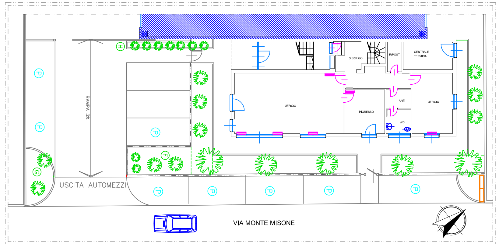
UFFICI MISIONE - PIANO TERRA
