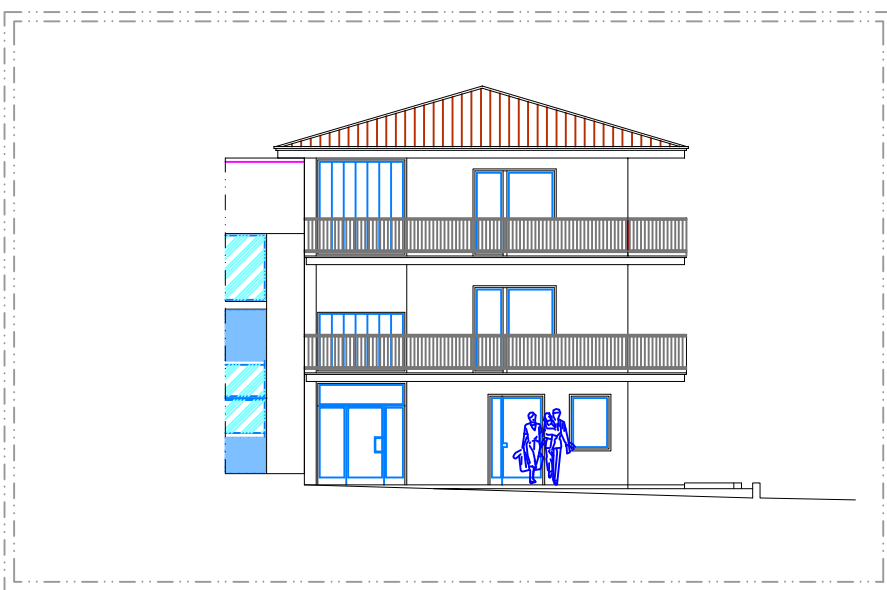
UFFICI MISIONE - PROSPETTO SUD
