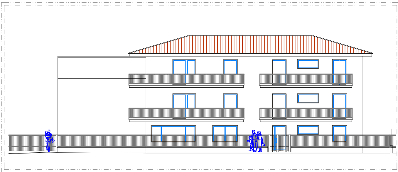
UFFICI MISIONE - PROSPETTO SUD
